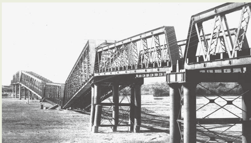
長良川(岐阜一穂積)鉄橋崩落
