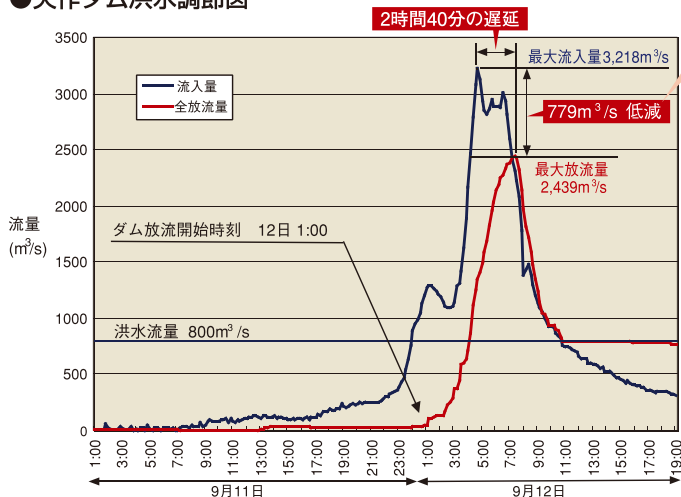
矢作ダム放流状況
