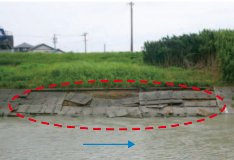
菊川左岸5.4kmの護岸が崩壊 出典：国土交通省 中部地方整備局 河川部
