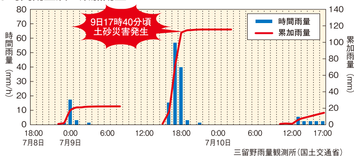
長野県木曽郡南木曽町梨子沢の土砂災害状況
