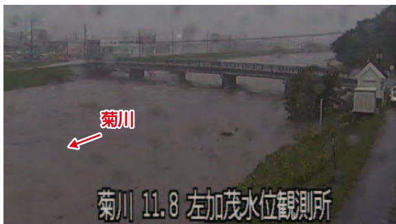
加茂水位観測所付近 出水状況(10月12日17時00分)
