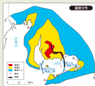
●震度分布図
