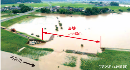
石沢川左岸1.0km付近の堤防決壊(秋田県由利本荘市) 出典：国土交通省 東北地方整備局 河川部
