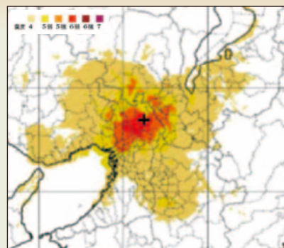
○推計震度分布図
