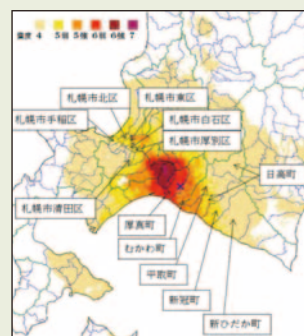
○推計震度分布図
