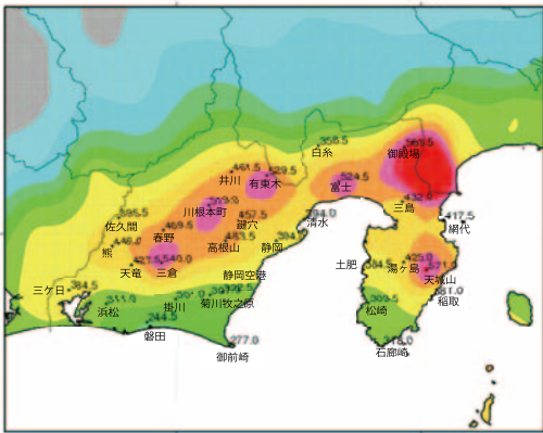
アメダス 降水量(mm) 出典:静岡地方気象台
