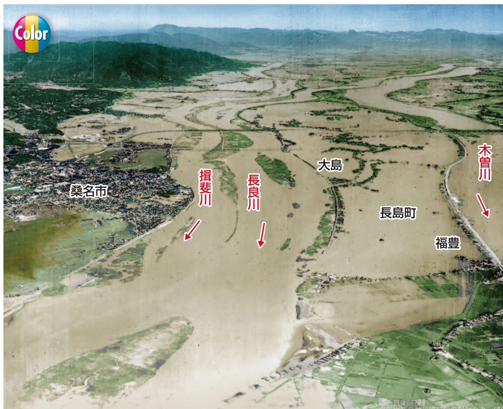
木曽三川下流域の浸水状況(長良川、揖斐川河口付近空から上流側を望む)
